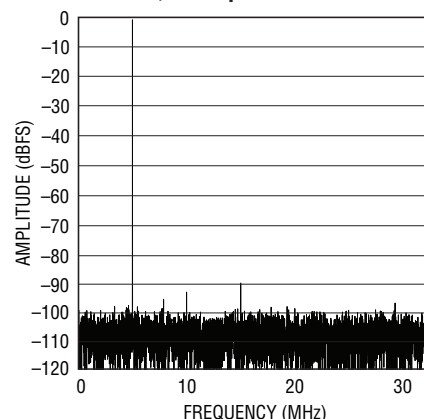
LTC2265-12: 8k Point FFT, f_{IN} = 5\text{MHz} , -1\text{dBFS} , 65\text{Msps}
