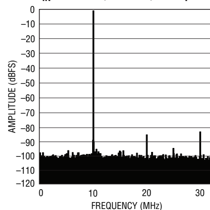
LTC2265-12: 8k Point FFT, f_{IN} = 140\text{MHz} , -1\text{dBFS} , 65\text{Msps}
